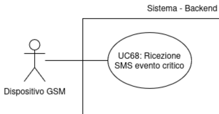
Figura 72: UC68 - Ricezione SMS evento critico
