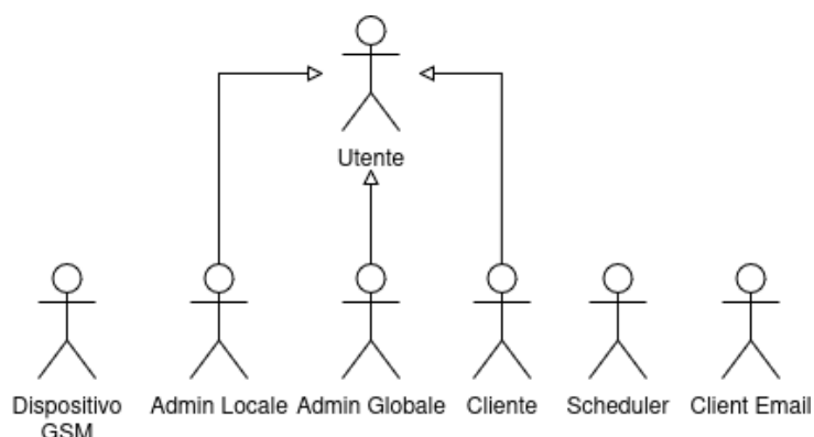
Figura 1: Diagramma degli attori principali
