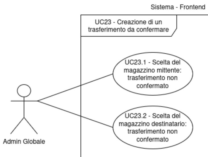
Figura 22: Inclusioni del Caso d'Uso n.23: UC23.1 e UC23.2
