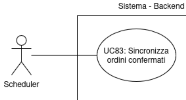
Figura 88: UC83 - Sincronizza ordini confermati
